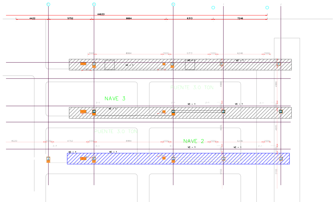
PLANTA CIMENTACION
